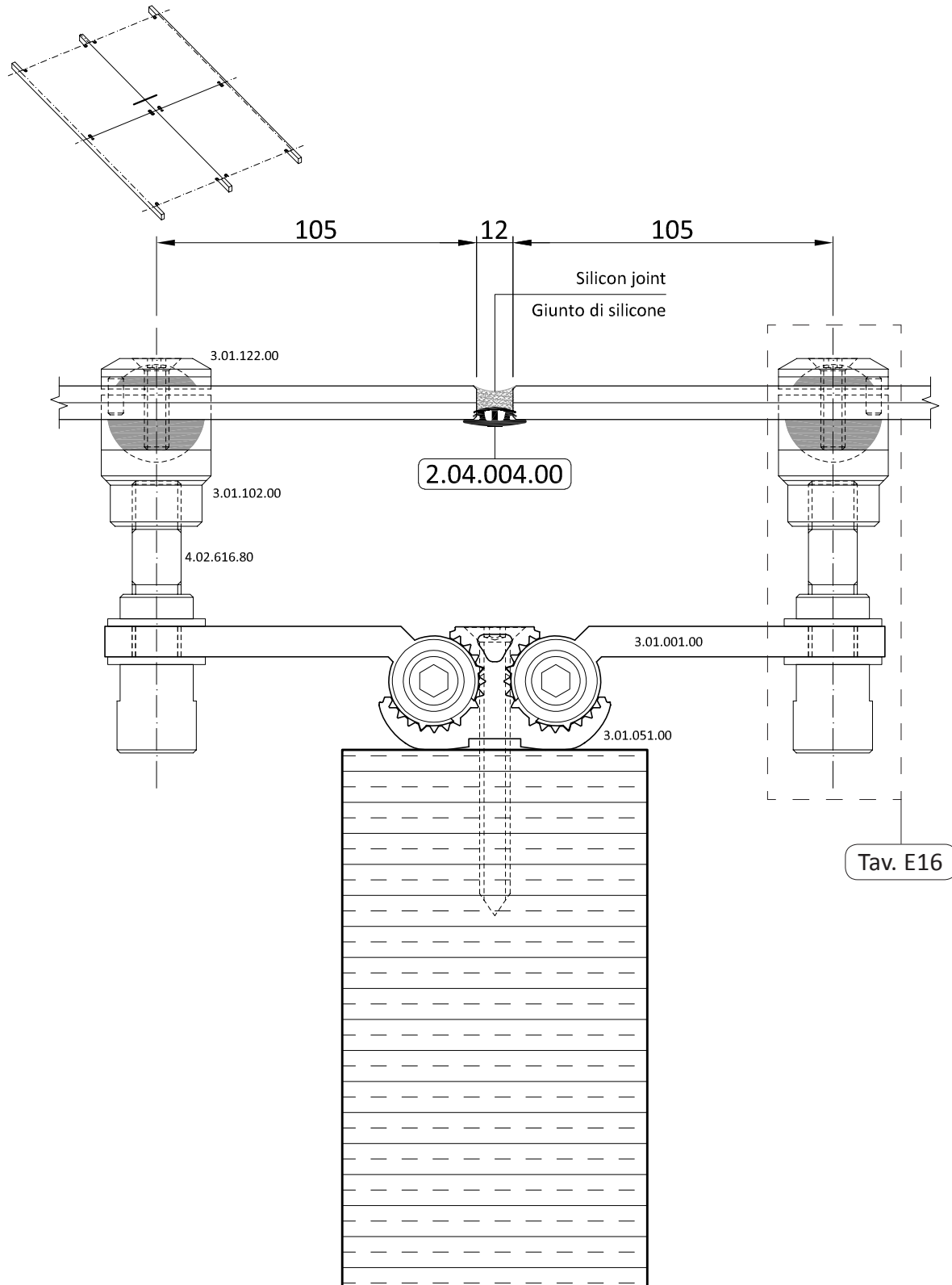
Tavola S61. Staffe orientabili su struttura portante in legno Table S61. Adjustable brackets on wood carrying frame
